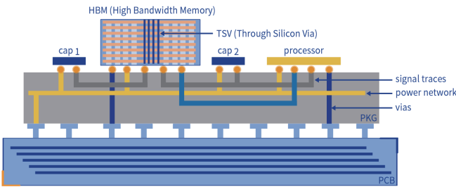
芯片、封装和 PCB 级信号完整性设计
